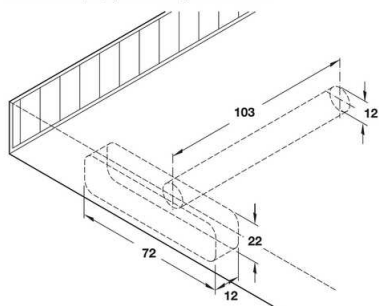
Dimensions de perçage et de fraisage dans la tablette
